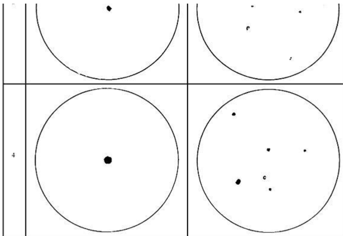
ШКАЛА N 4 КАРБИДНАЯ СЕТКА × 500
